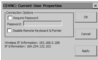
Figura 5.10: Escritorio Remoto
